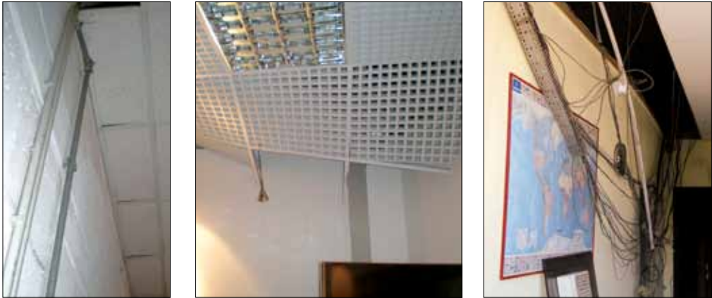
Figura 6.15: Esempi di danni ad elementi non strutturali secondari: (a) danno ad elementi di una controsoffittatura ispezionabile; (b) collasso di una controsoffittatura; (c) collasso di elementi in cartongesso di una controsoffittatura ispezionabile (terremoto Emilia-Romagna 2012, Mirandola (MO))
